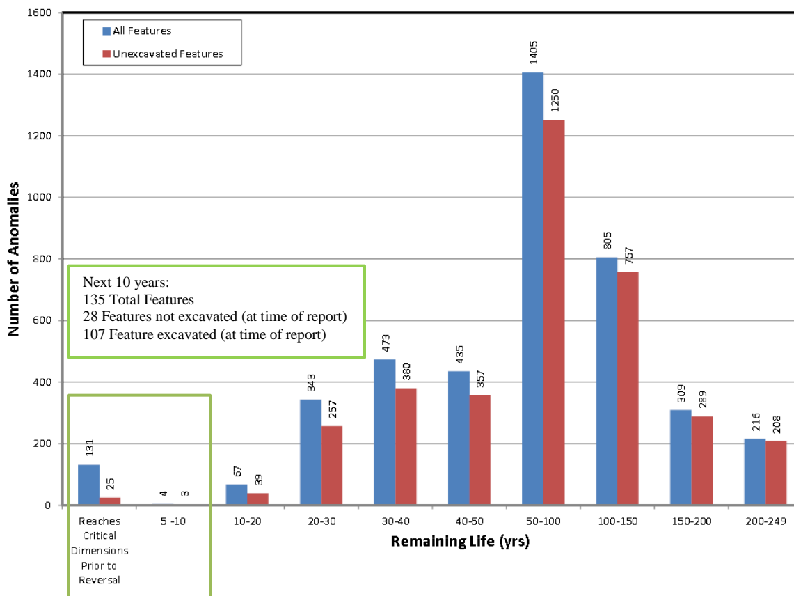
Figure 4.46 – Évaluation déterministe de la durée de vie restante des éléments détectés par la DFUS (du PNW au TM)
